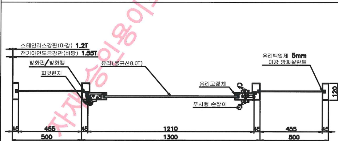
제품 A-A' 상세도
